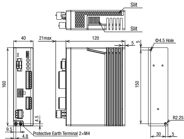
RKSD503-A (M-A)
