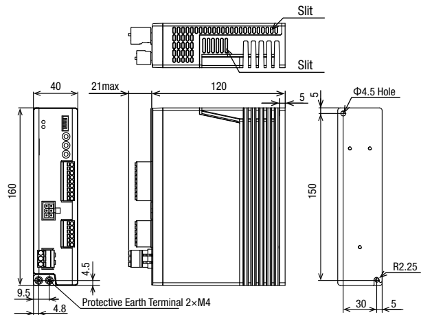
RKSD507-A (M-A)
